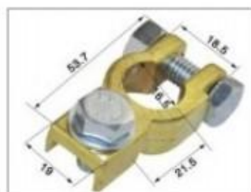
DJQ93085负极
