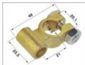
DJQ93083-35 2 负极
